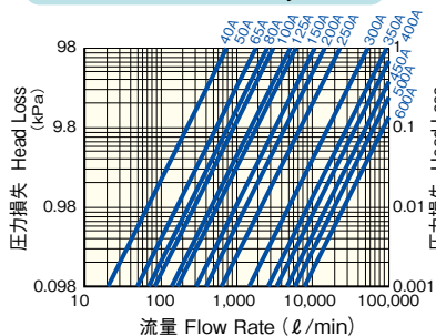
バタフライバルブ Butterfly Valve
