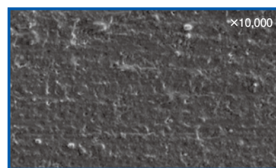
通常の塩ビ管 Ordinary U-PVC Pipe
