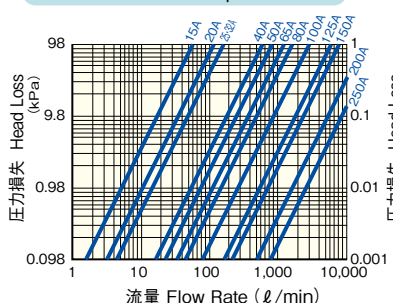
ダイヤフラムバルブ Diaphragm Valve
